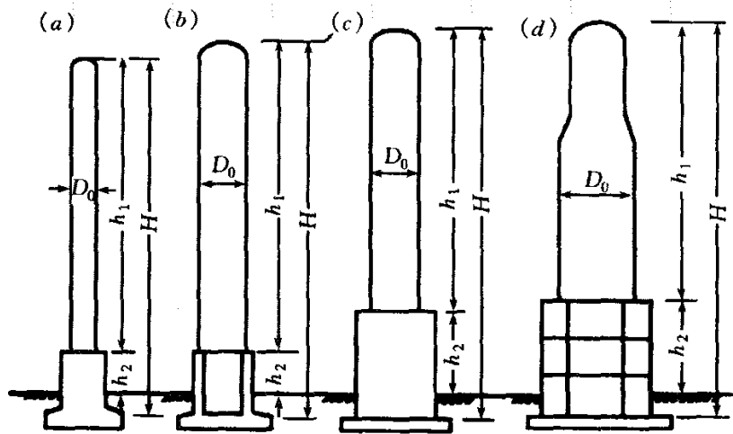
图 E.1.2 设备塔架的基础型式 (a) 圆柱基础塔; (b) 圆筒基础塔; (c) 方形 (板式) 框架基础塔; (d) 环形框架基础塔
