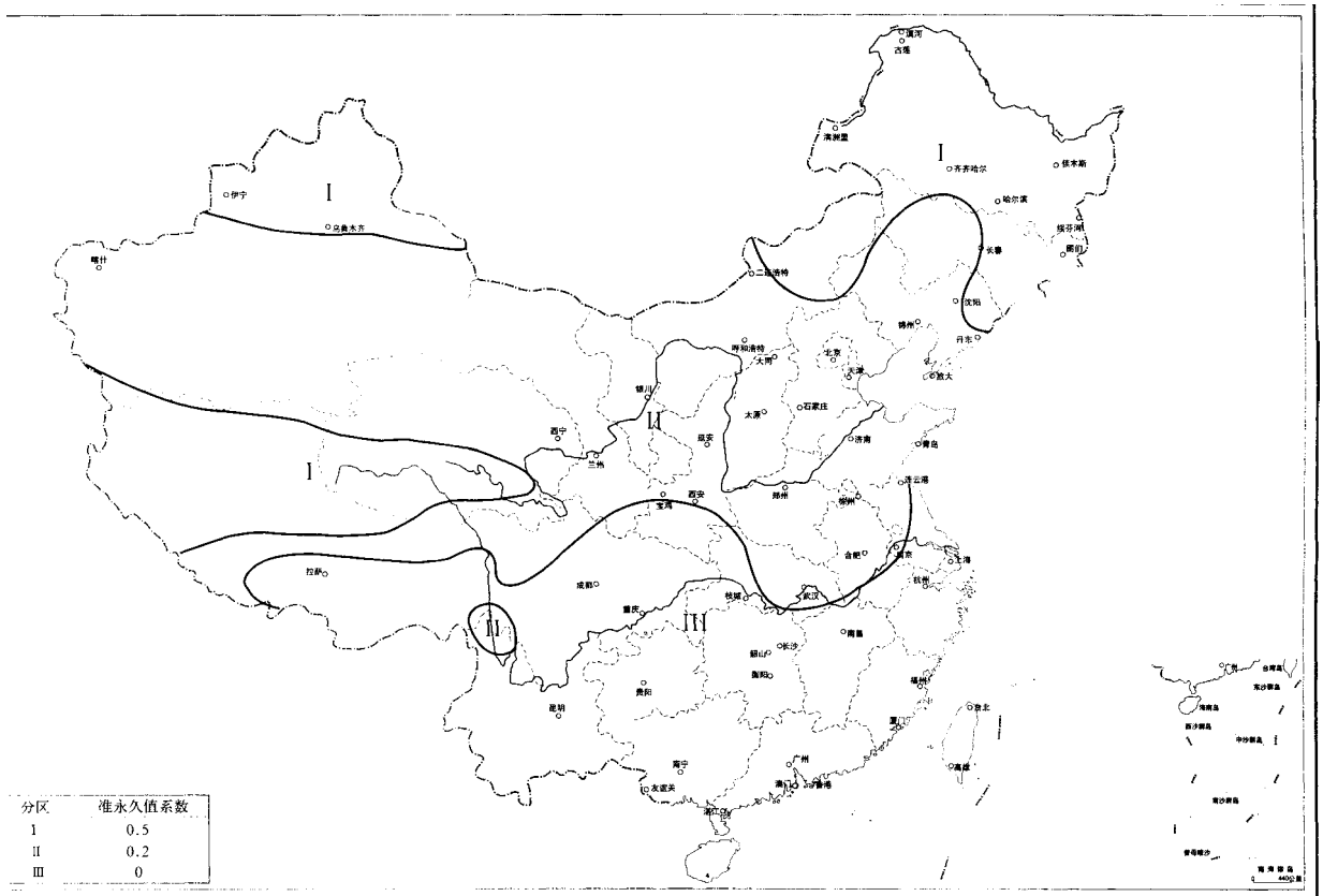
附图 D.5.2 各荷载准永久值系数分区图
