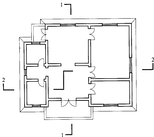
图 4.3.4 剖切符号
