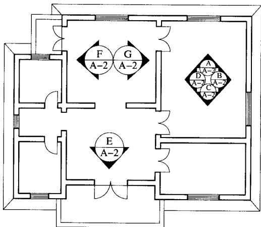
图 4.1.8-3 平面图上内视符号(带索引)应用示例
